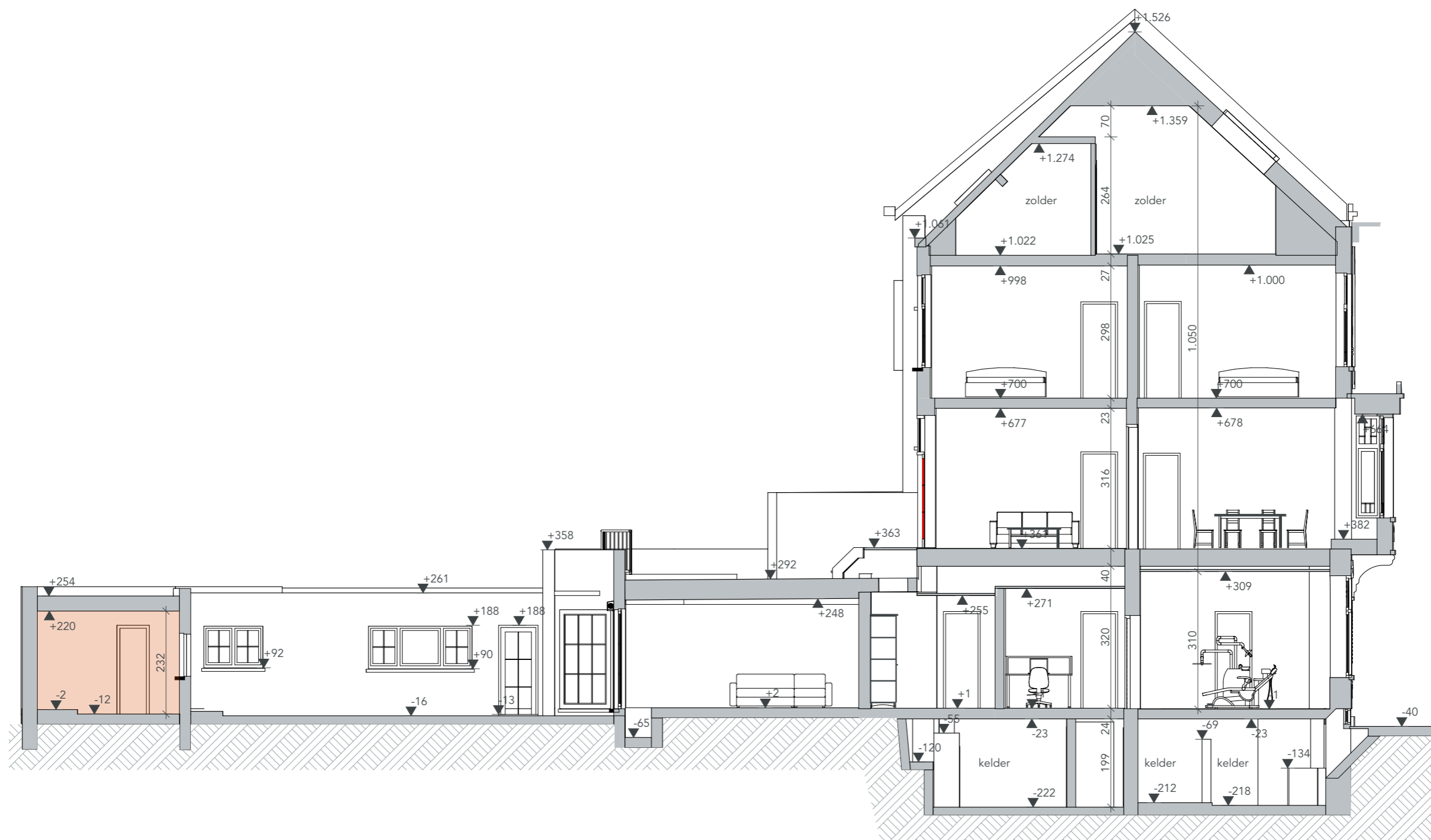
0 1 2 3 4 BT Langsdoorsnede AA'
