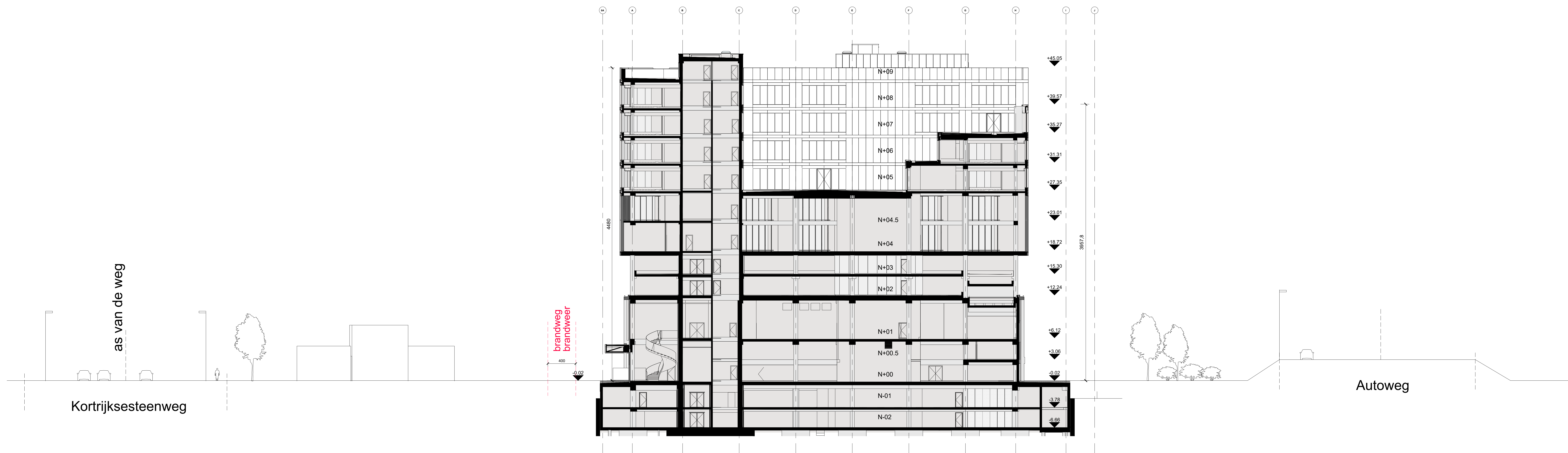
Terreinprofiel schaal 1/200
