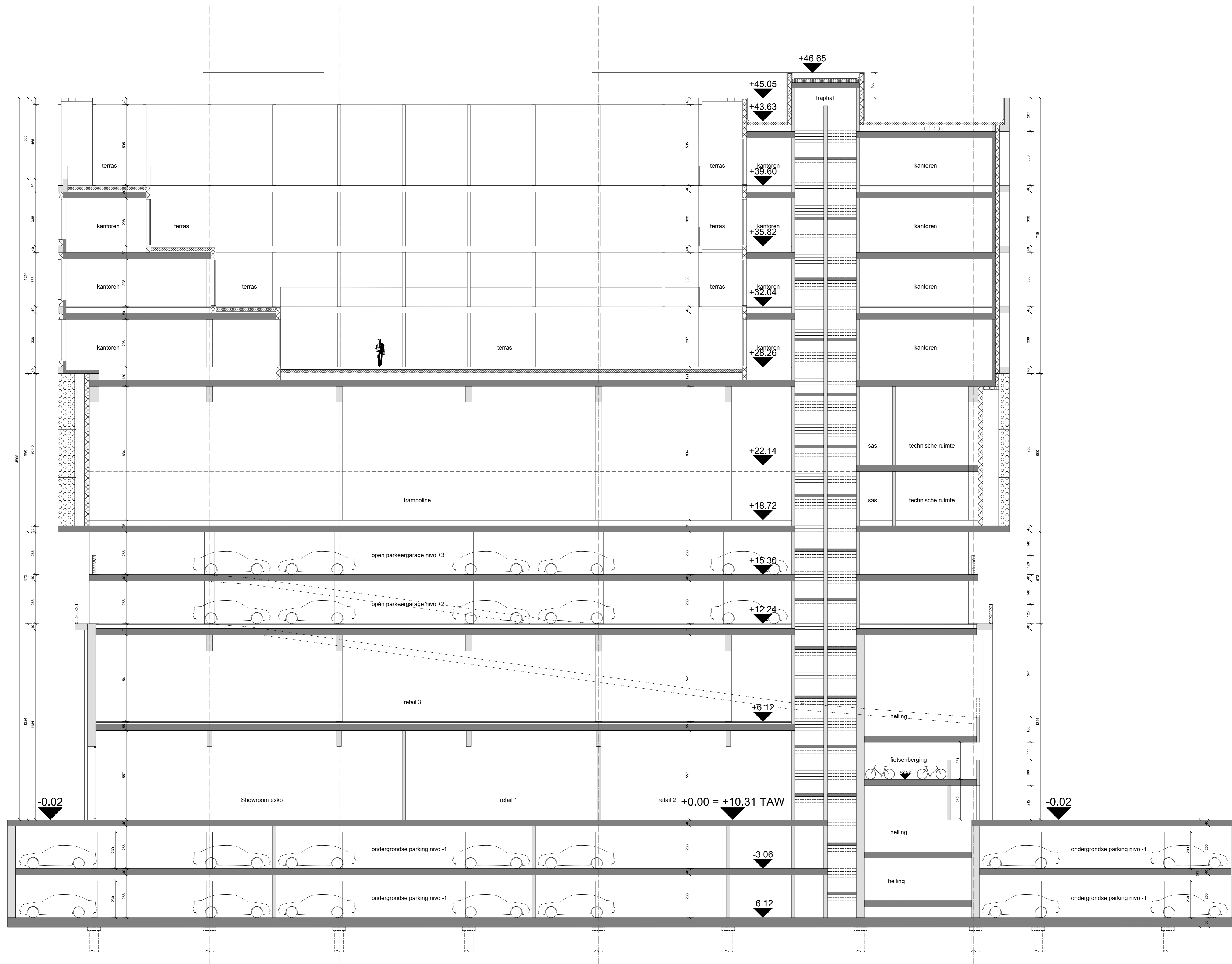
Doorsnede AA
