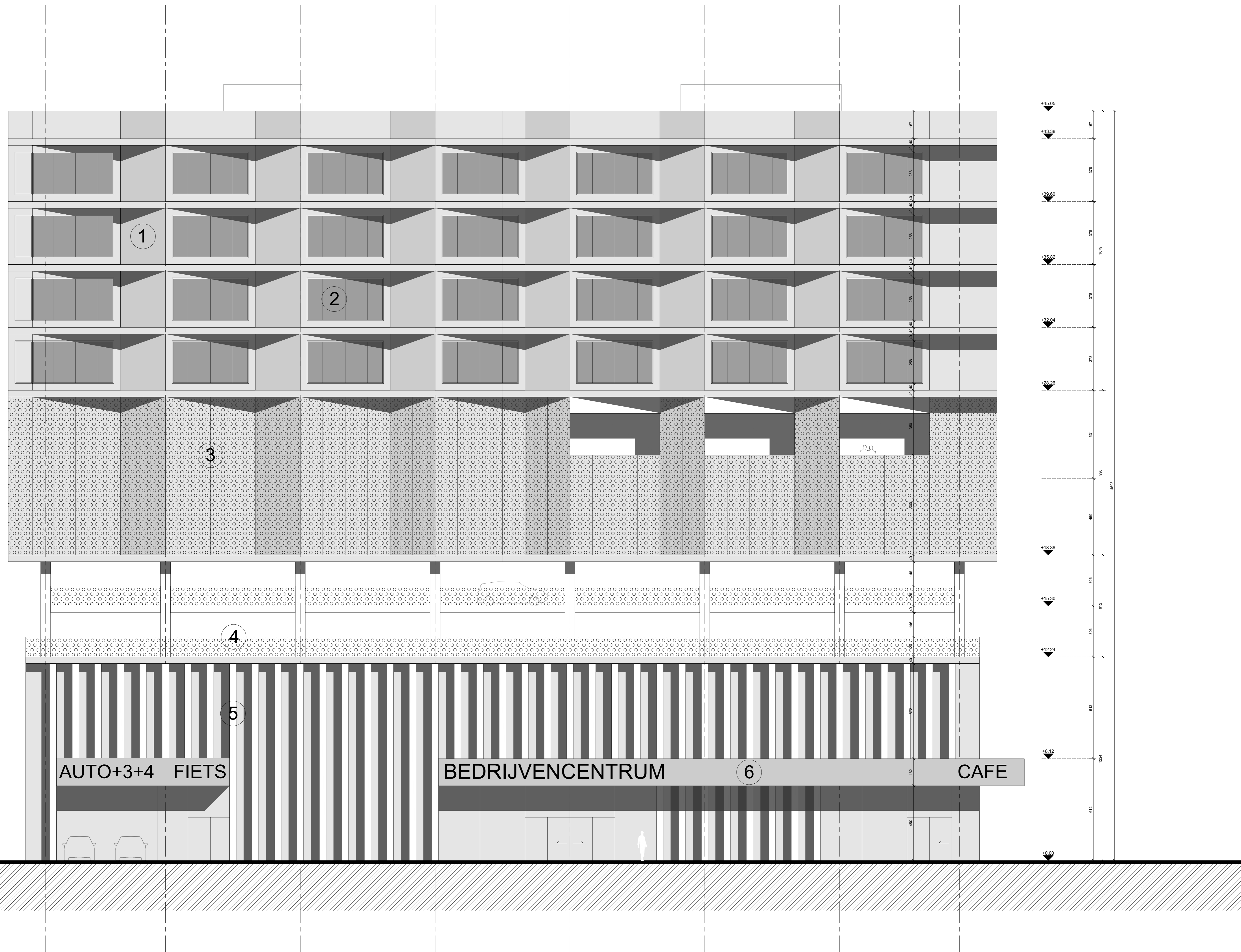
Gevel Noord - West schaal 1/100
