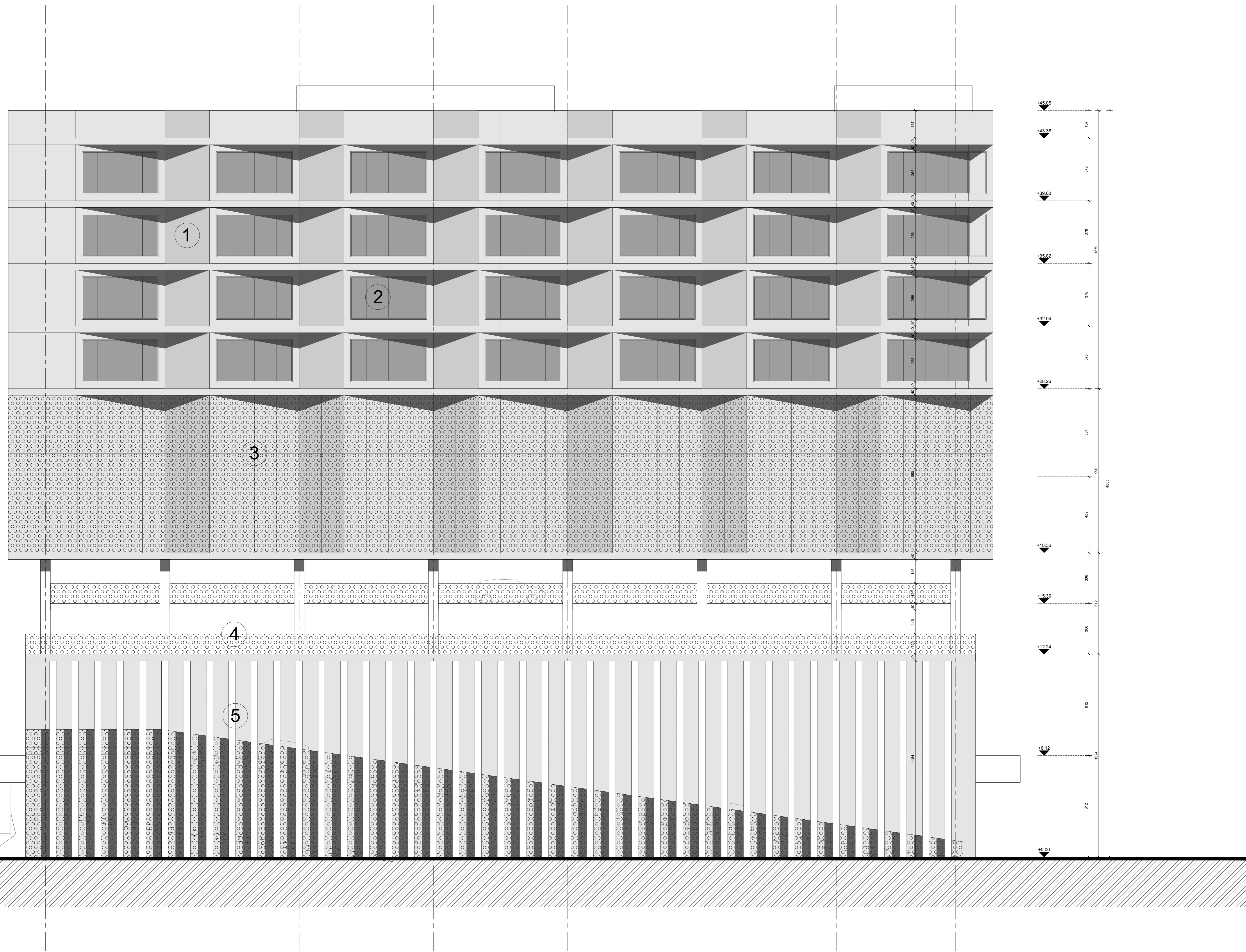
Gevel Noord - Oost schaal 1/100
