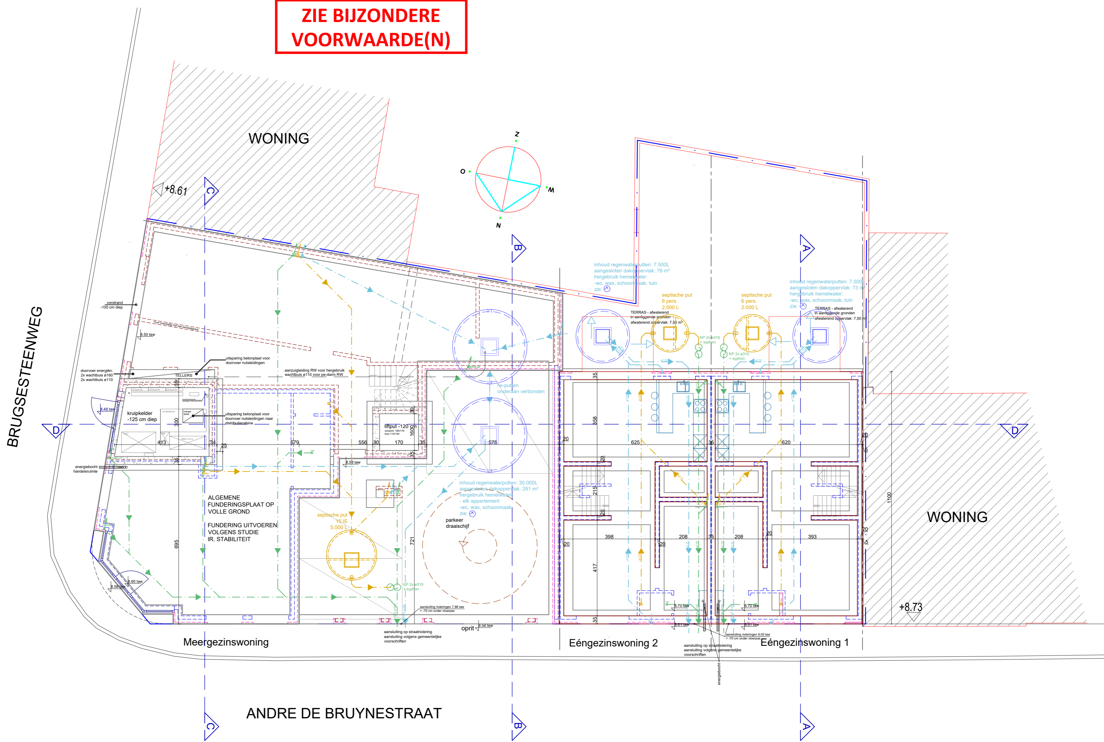
Funderings- en rioleringsplan 1:100
