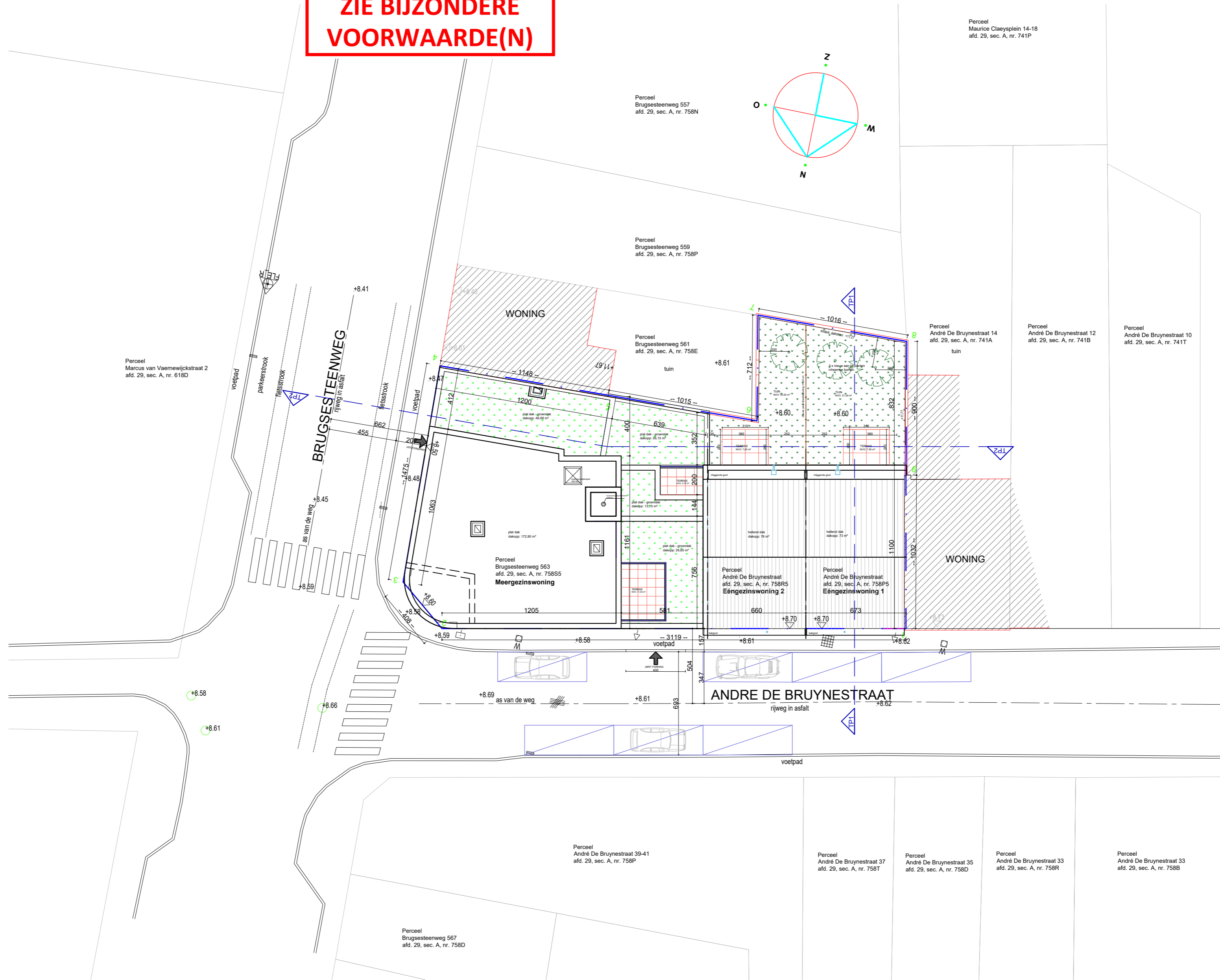
Inplantingsplan - nieuwe toestand 1:200
