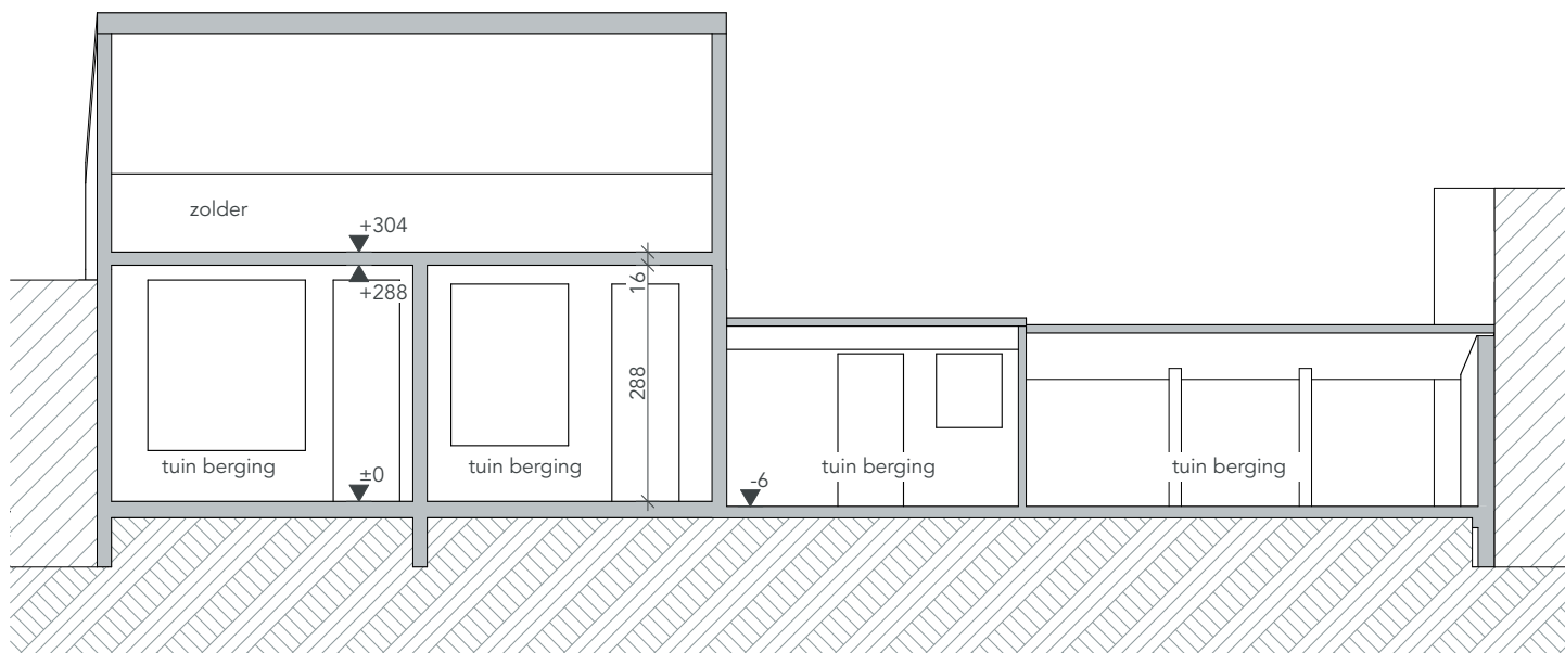
VT Doorsnede B-B
