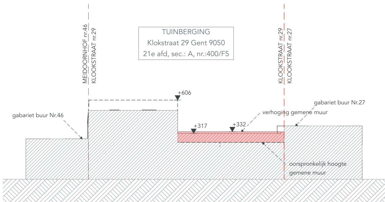
0 1 2 3 4 BT Terreinprofiel
