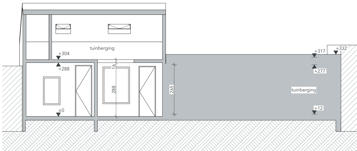
0 1 2 3 4 BT Doorsnede B-B
