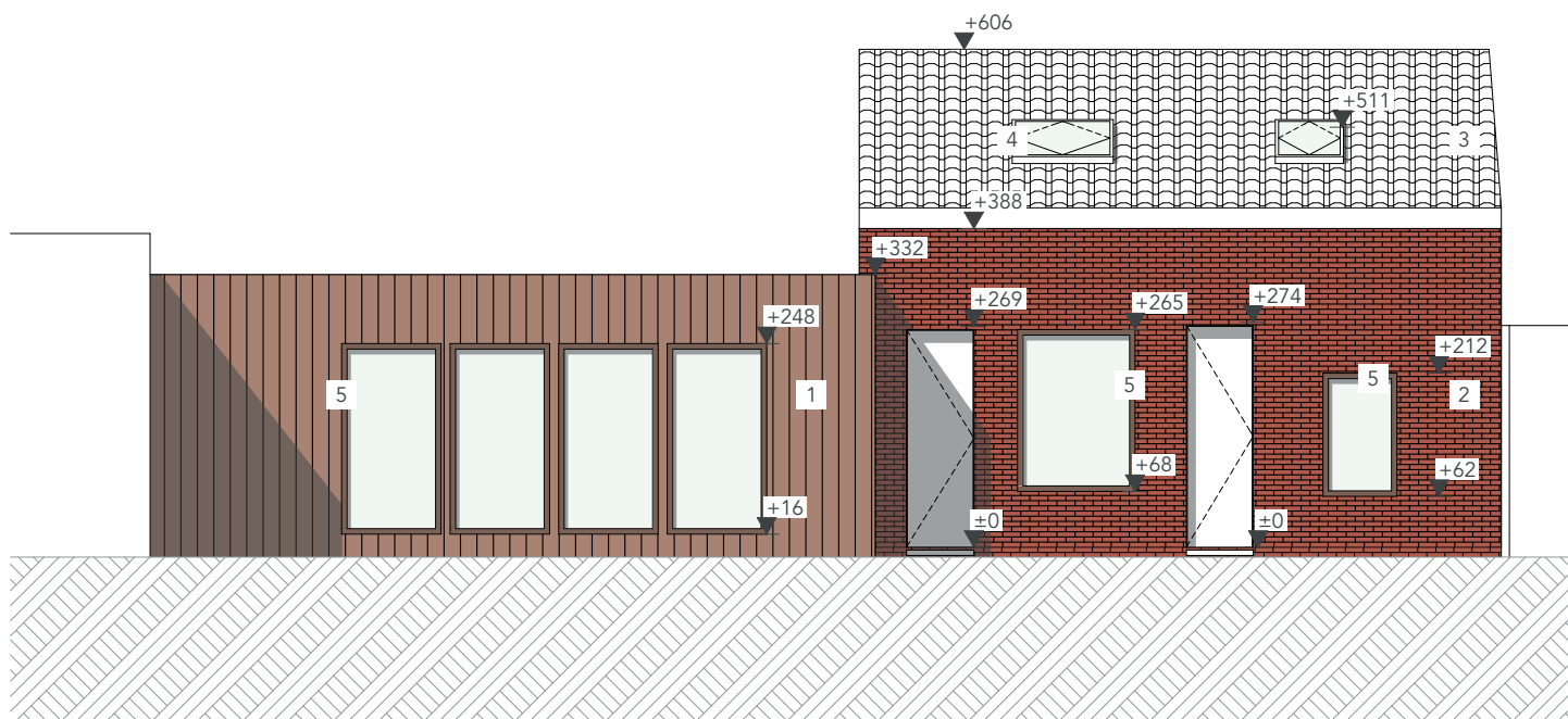
0 1 2 3 4 NT Rechtergevel
