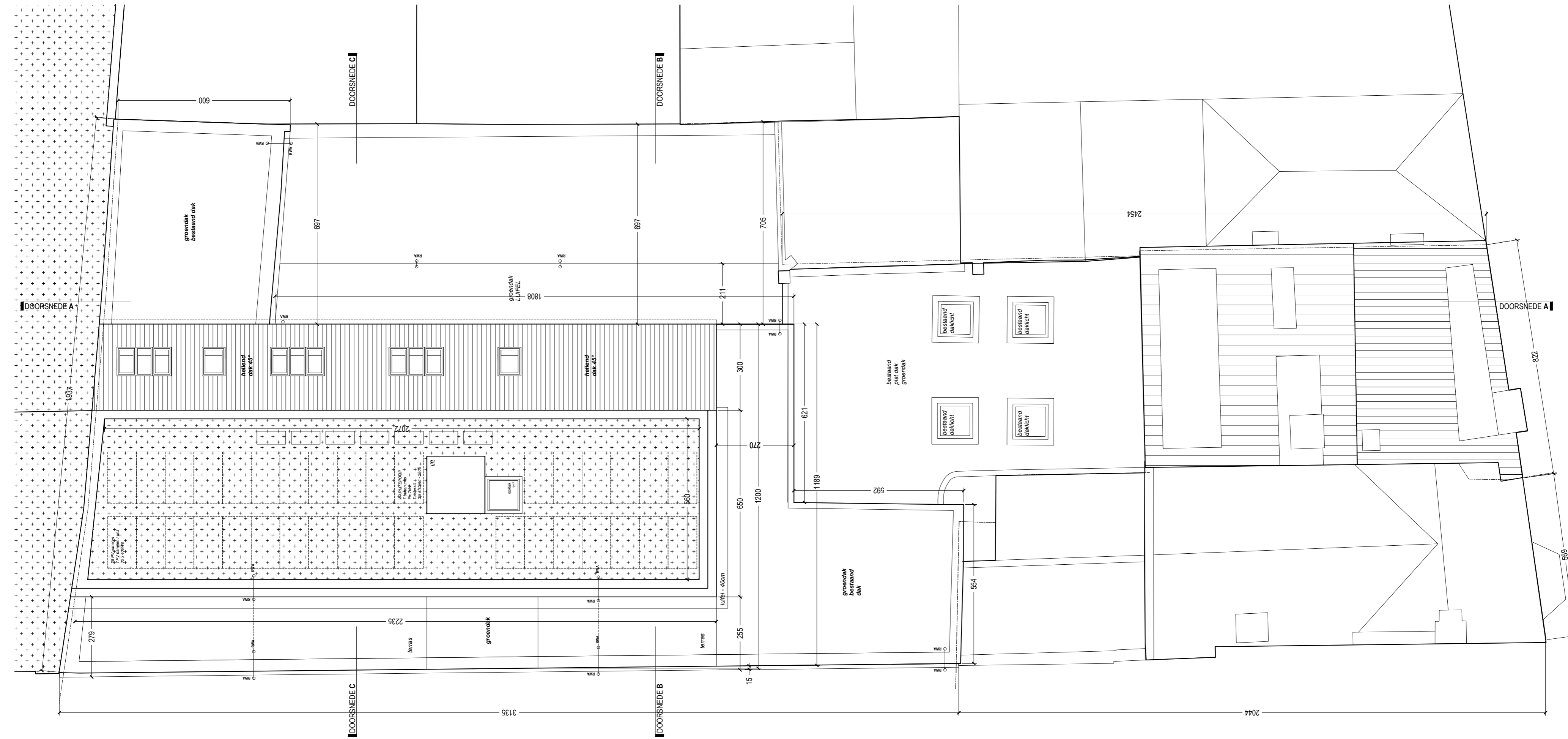
DAKENPLAN NIEUWE TOESTAND SCHAAL 1/100
