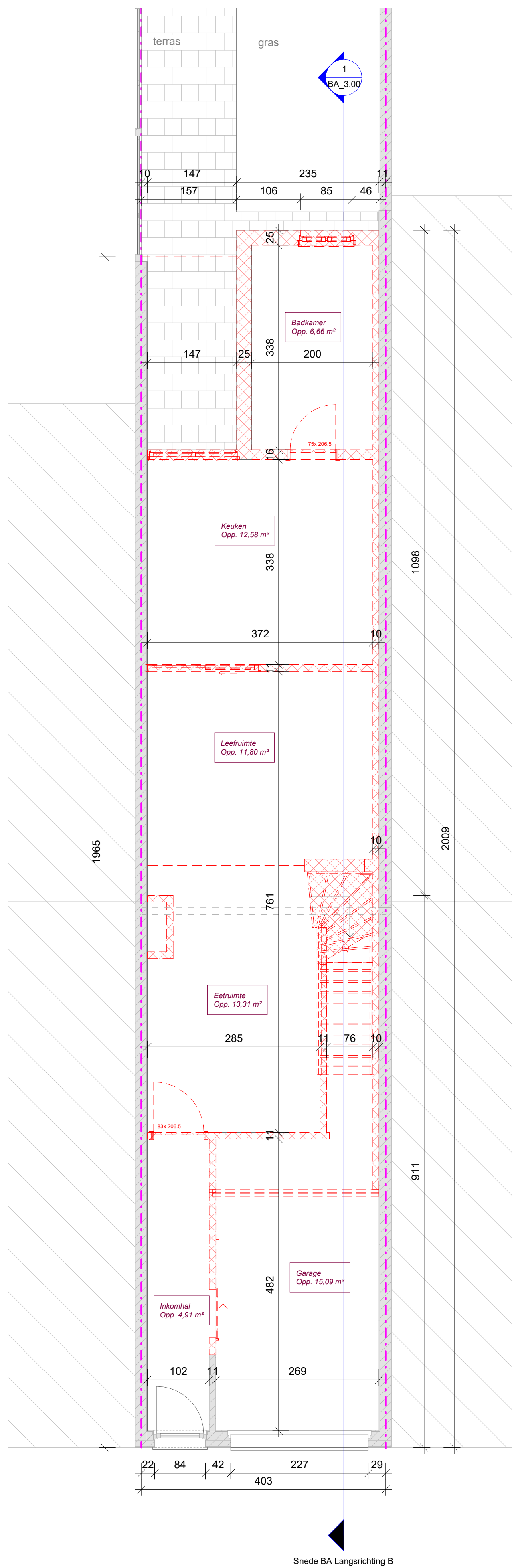
BA_1.00 P_B_1.00_Grondplan Gelijkvloers
