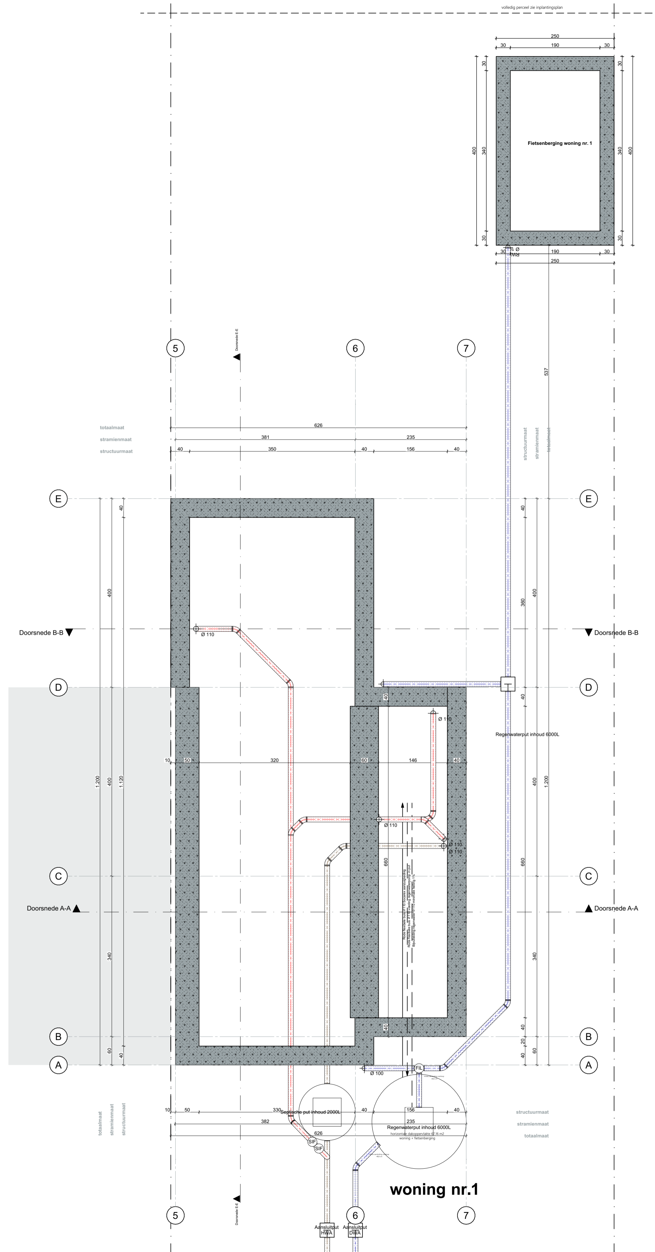
Funderings- en rioleringsplan, 1:50 Plattegronden Nieuwe toestand
