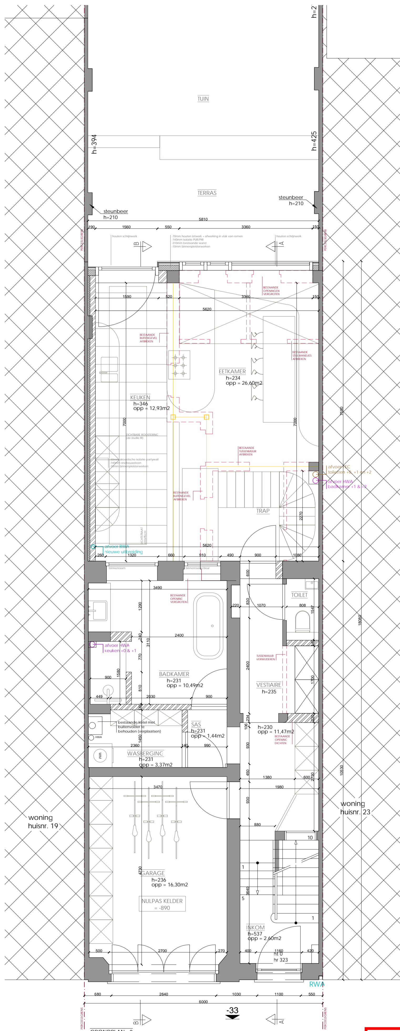
GRONDPLAN +0 nieuwe toestand schaal 1/50
