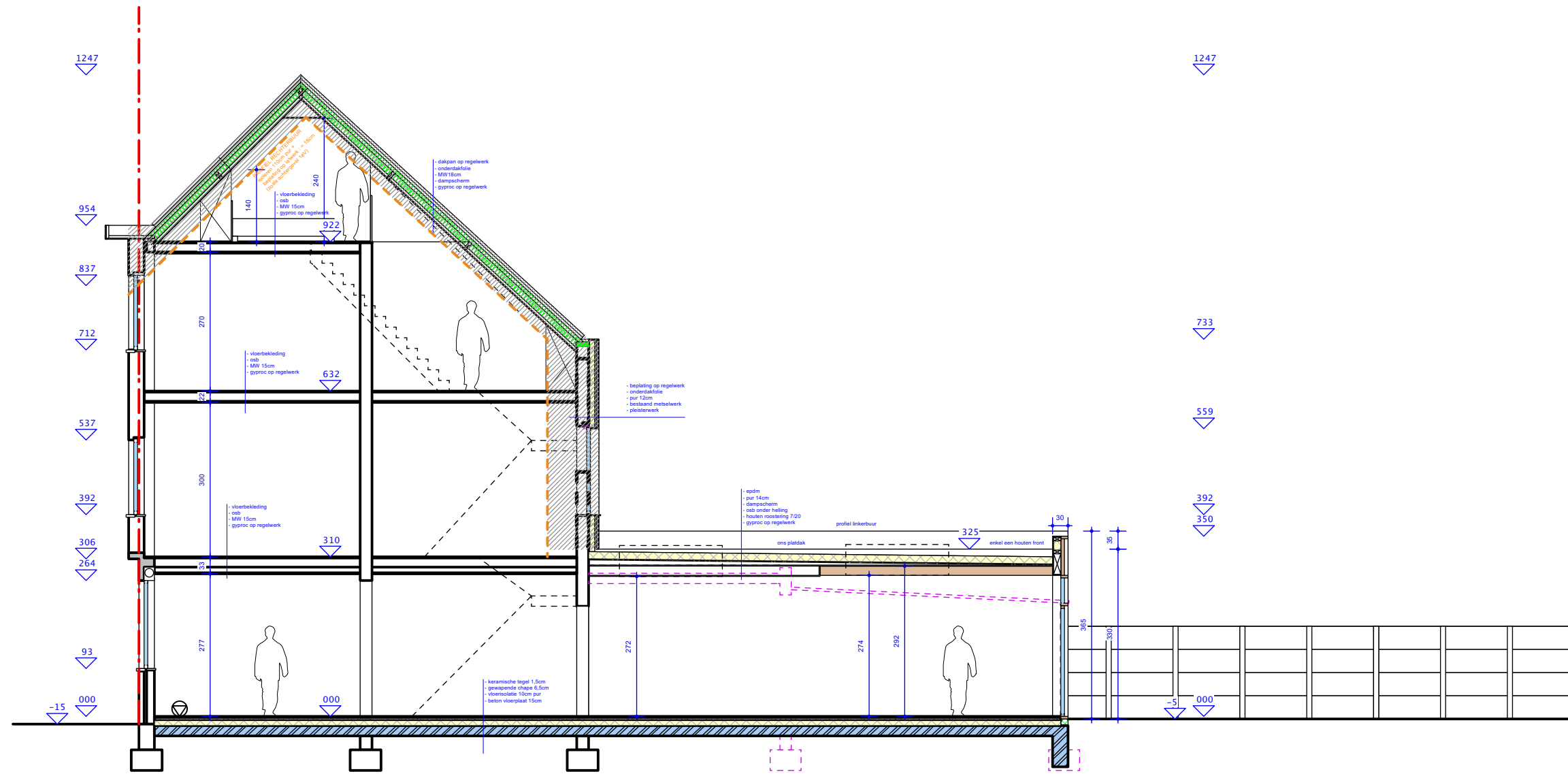
DOORSNEDE AA' (nieuw) 0 100 200 300 cm SCHAAL 1 / 100
