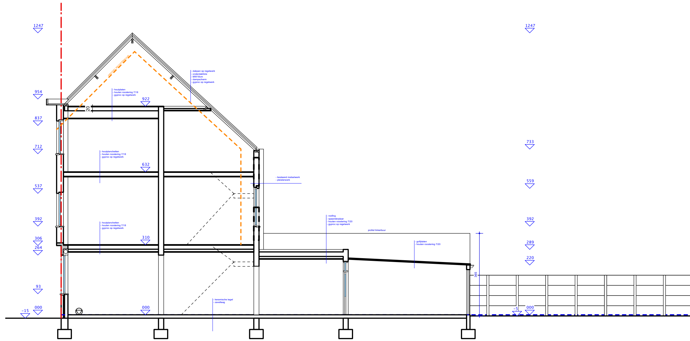
DOORSNEDE AA' (bestaande) 0 100 200 300 cm SCHAAL 1 / 100
