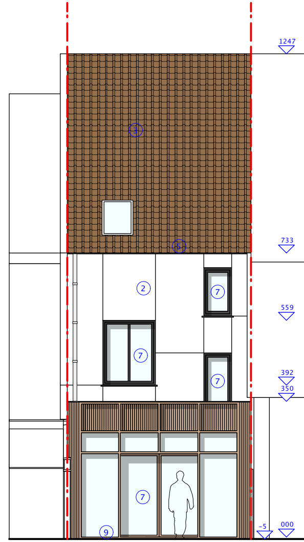
ACHTERGEVEL (nieuw)
