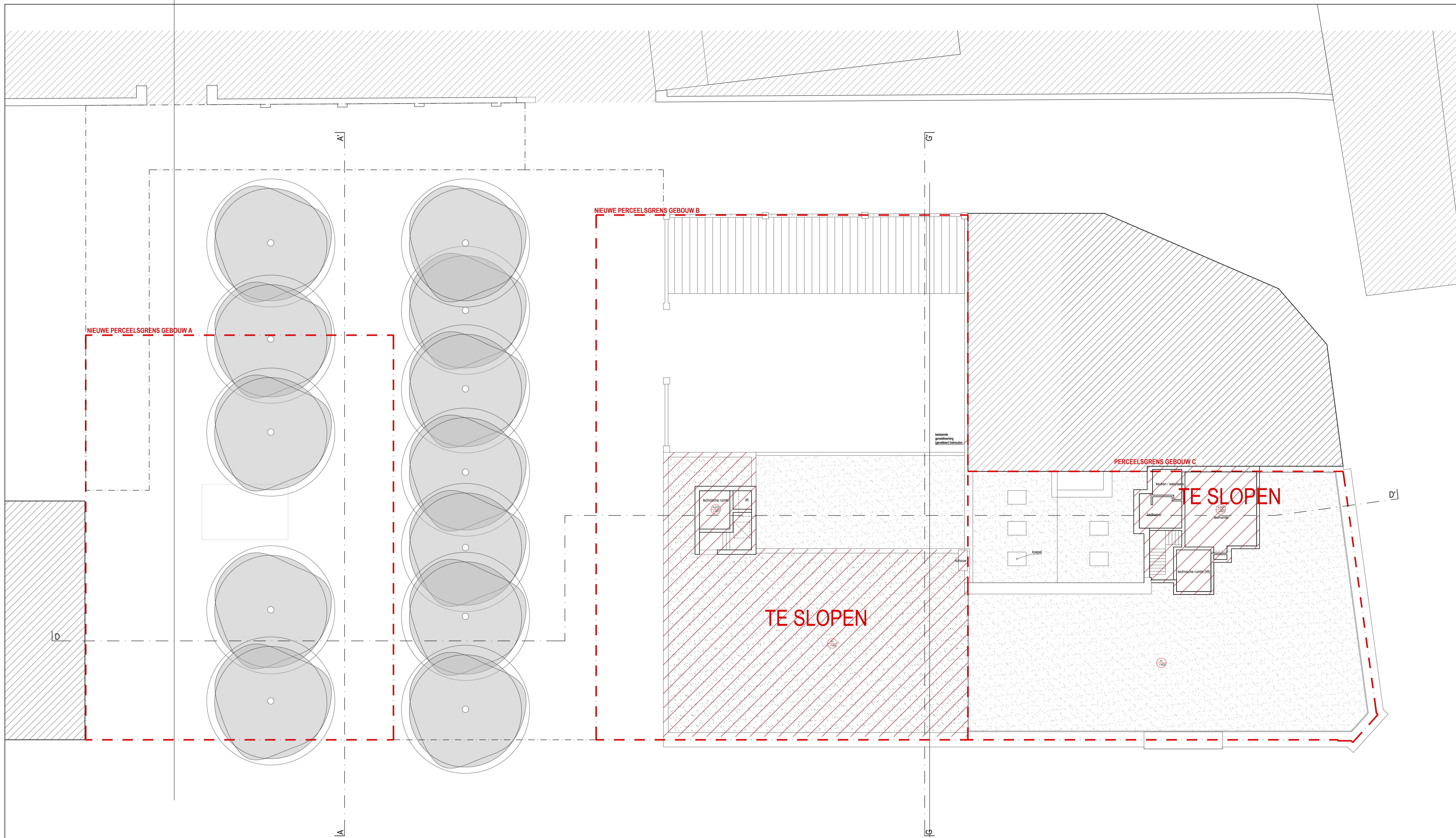
GRONDPLAN VERDIEPING +4 NIEUWE TOESTAND
