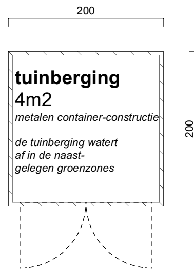
grondplan
