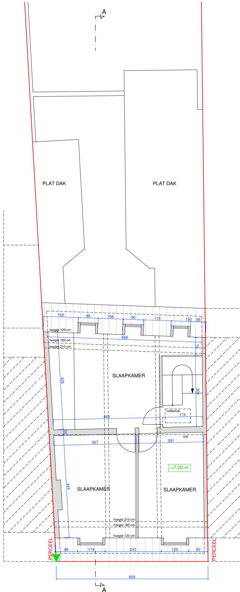
VERDIEPING 2 bestaande toestand
