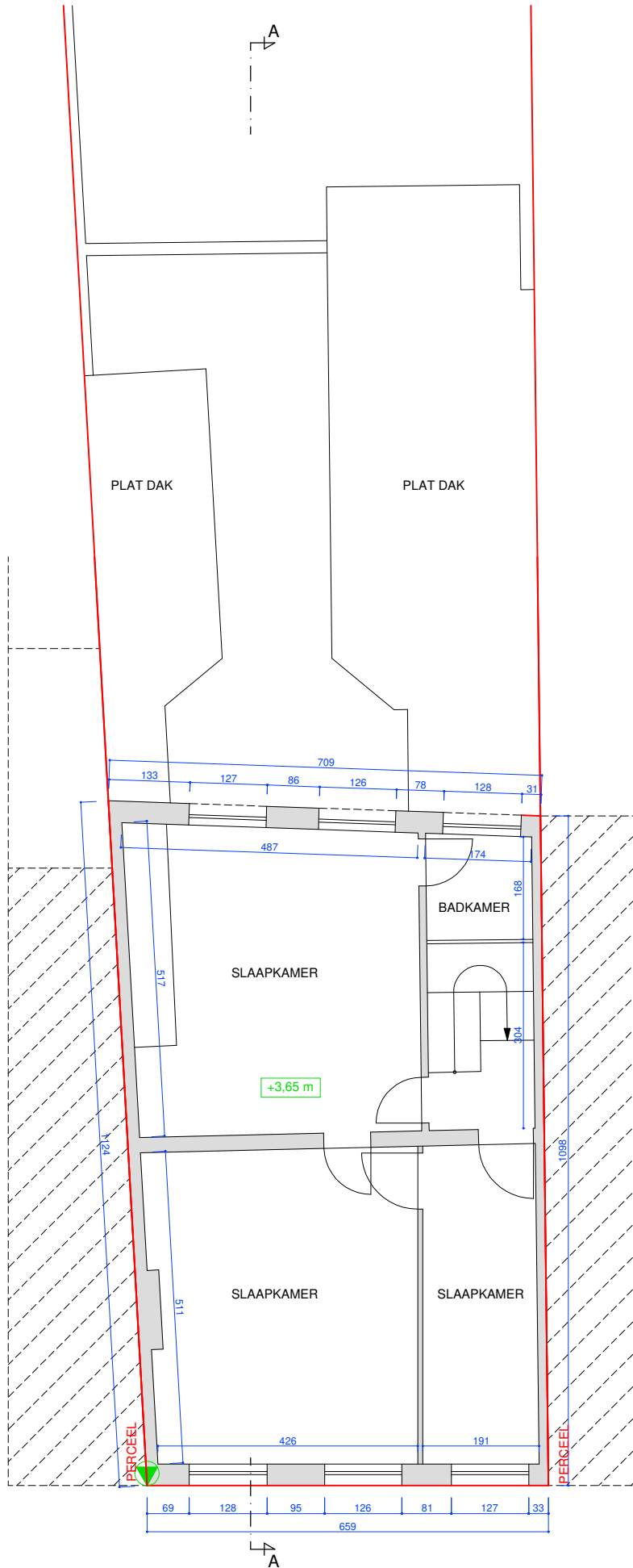
VERDIEPING 1 bestaande toestand
