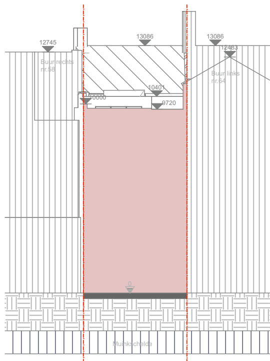
terreinprofiel dwars vergund 1:200
