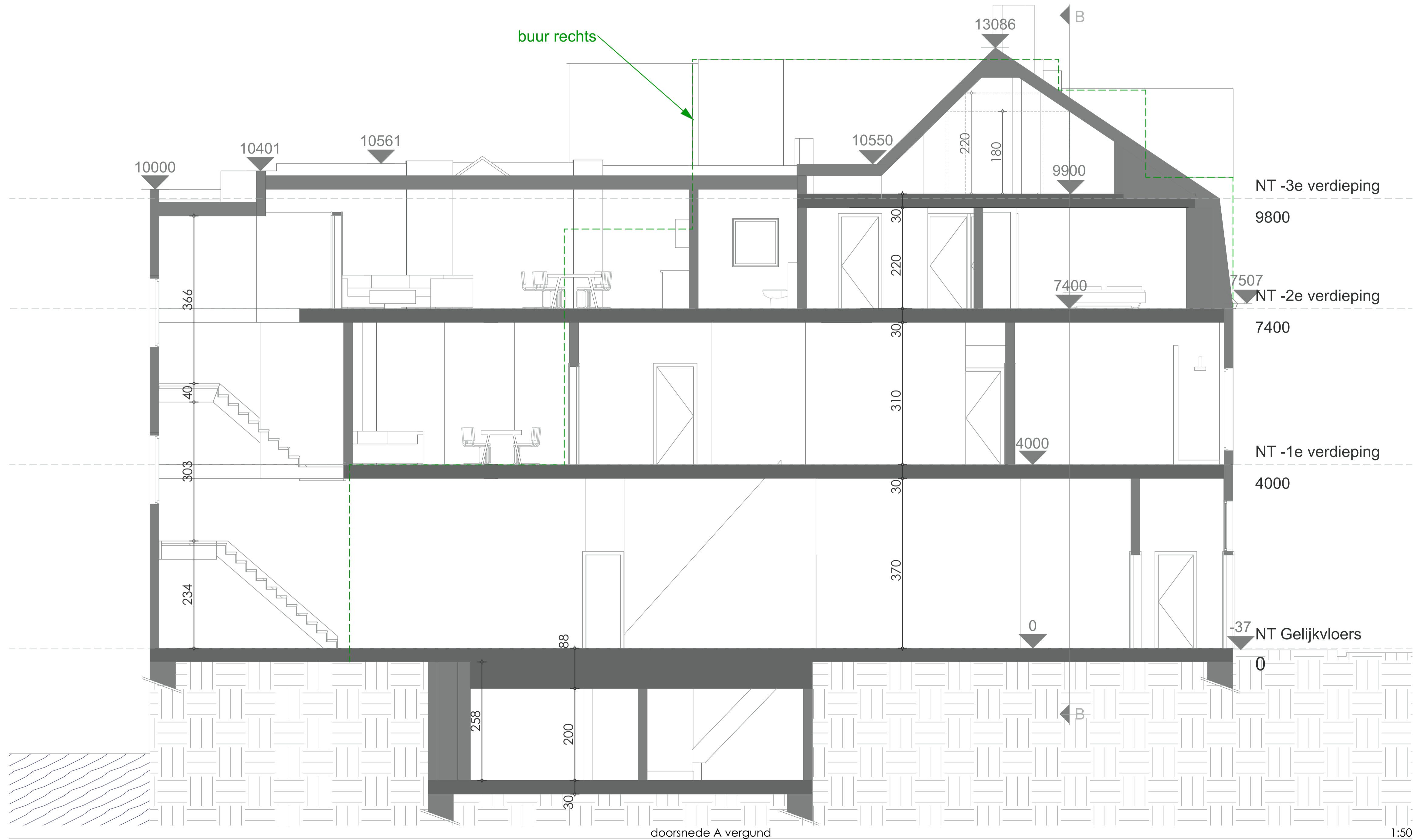
doorsnede A vergund
