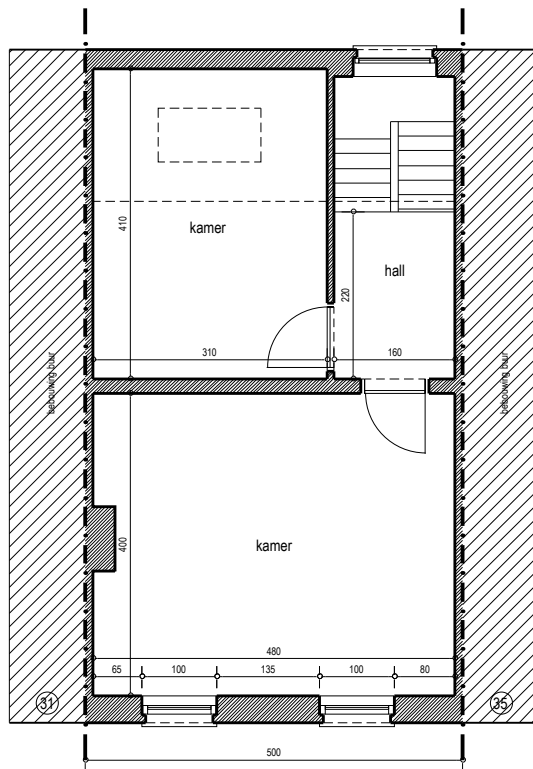
bovenverdieping bestaande toestand Raf Verhaeststraat 33
