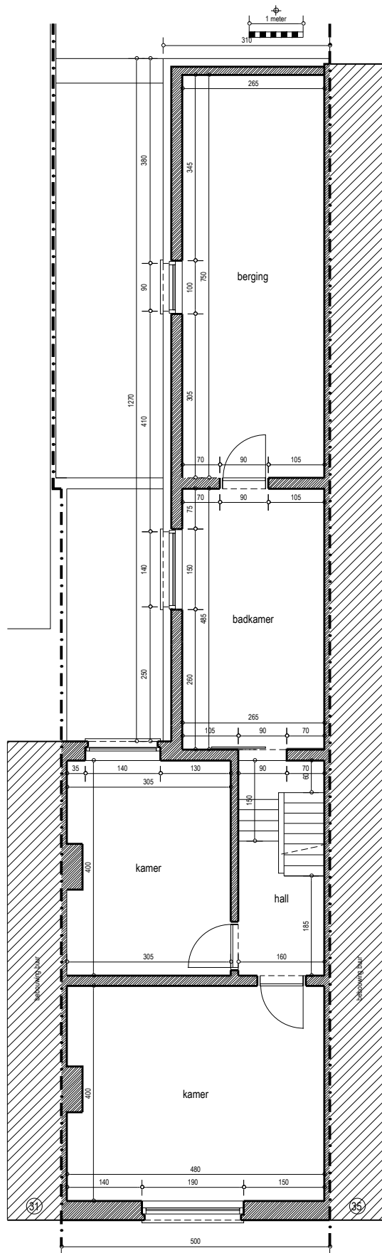
tussenverdieping nieuwe toestand Raf Verhaeststraat 33
