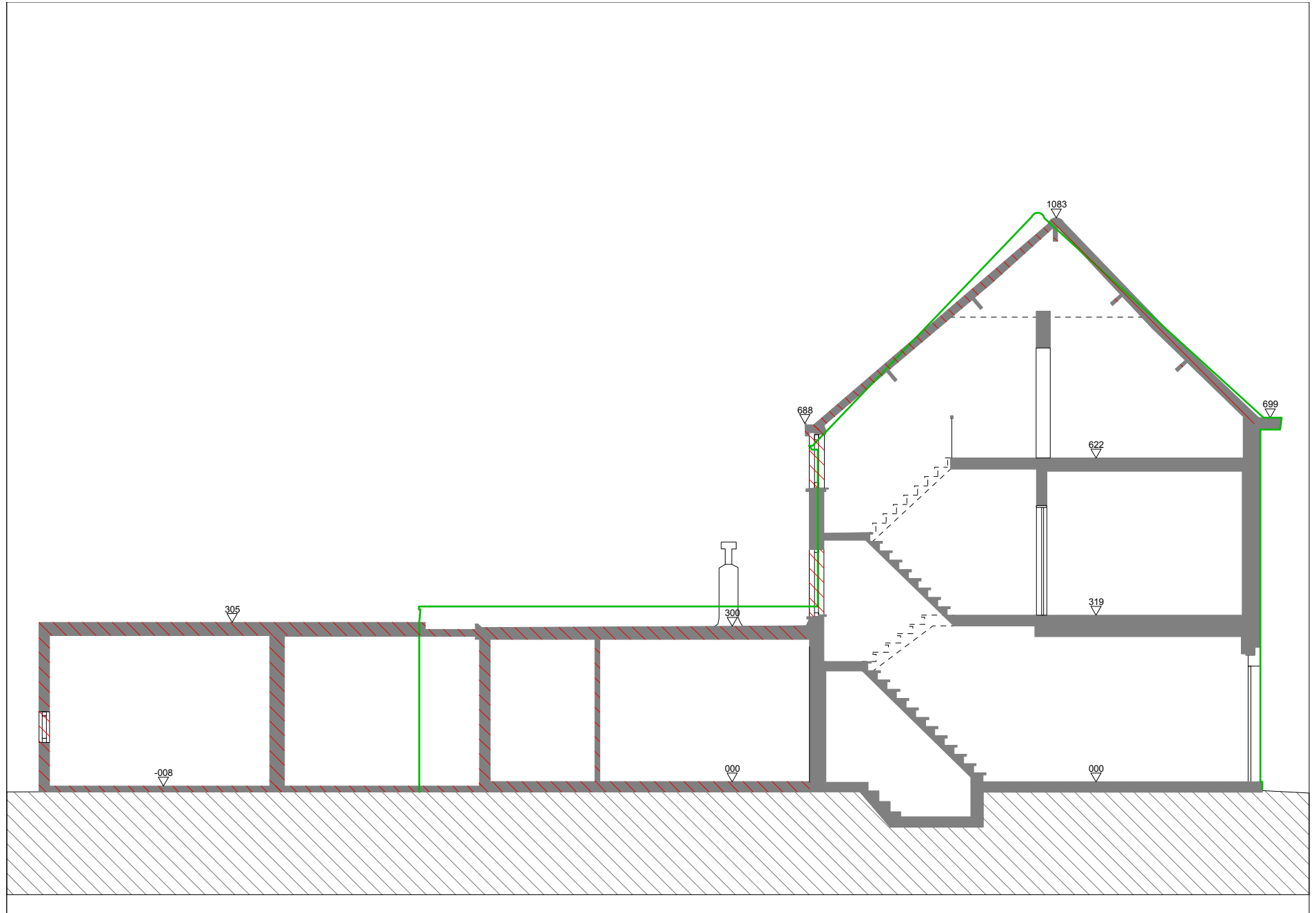
SNEDE BB' BESTAAND 1:100
