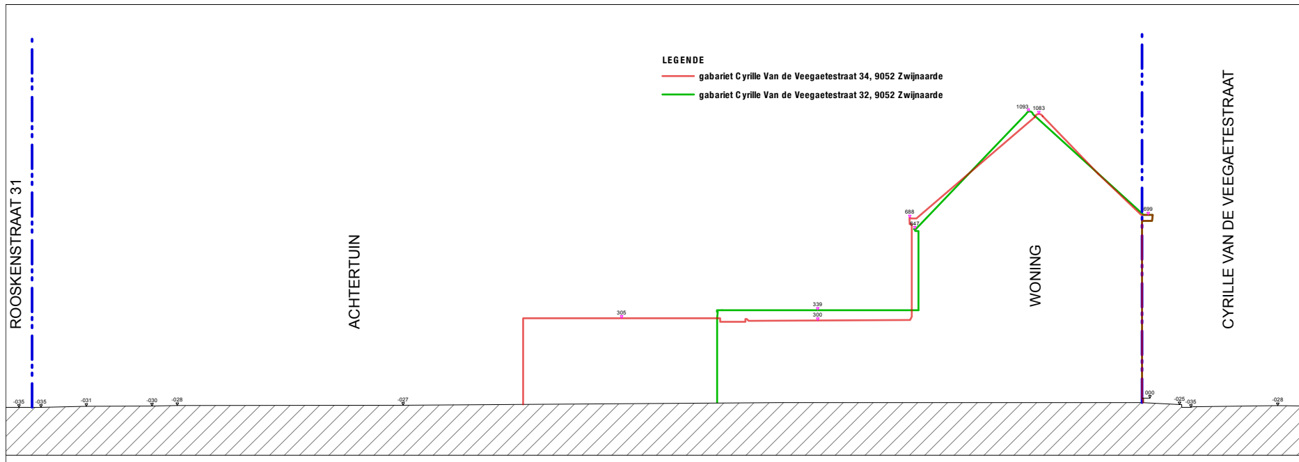
TERREINPROFIELEN BESTAAND 1:200
