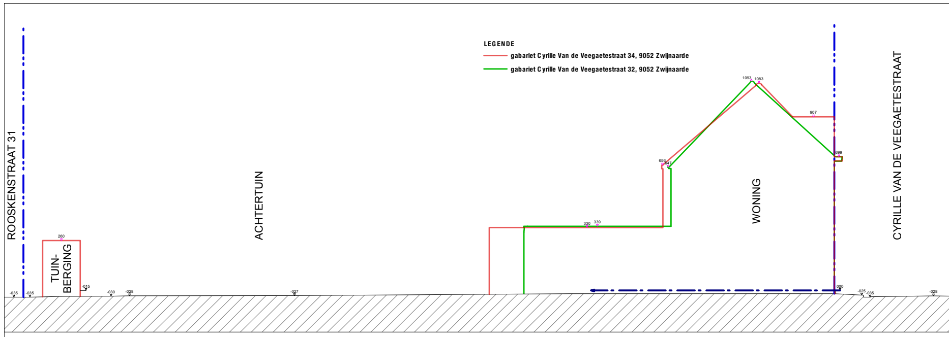
TERREINPROFIELEN NIEUW 1:200
