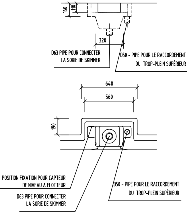
DETAIL SKIMMER INTÉGRÉ M 1:25
