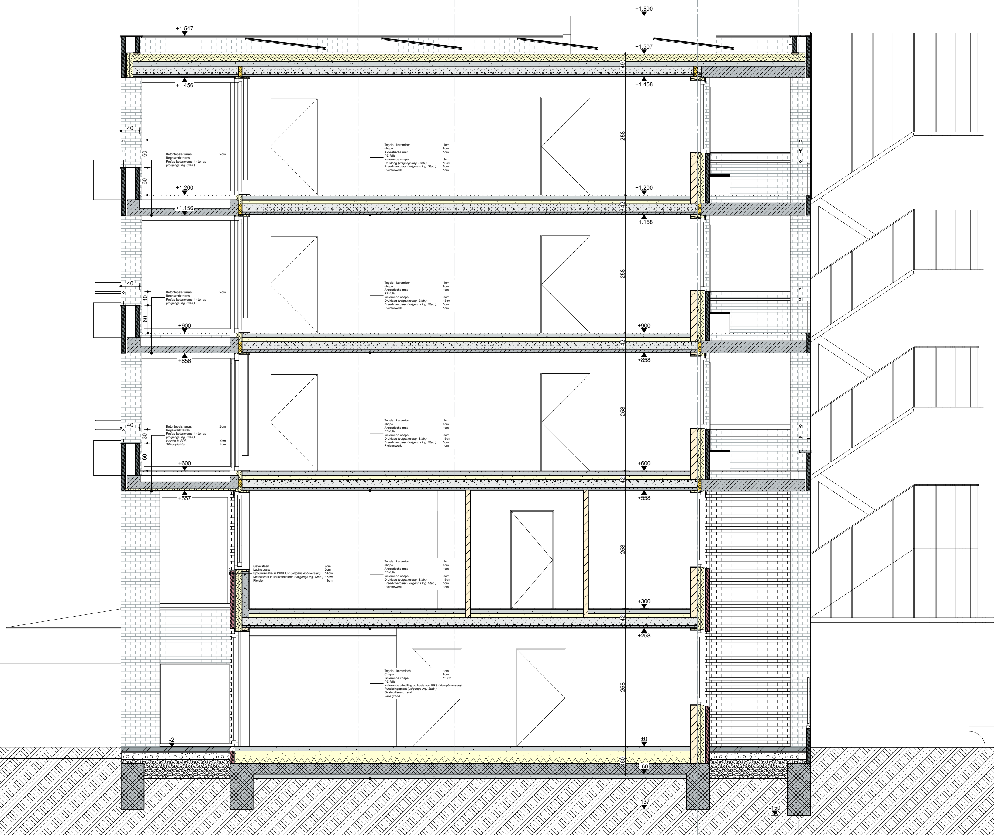
Doorsnede H-H NT
