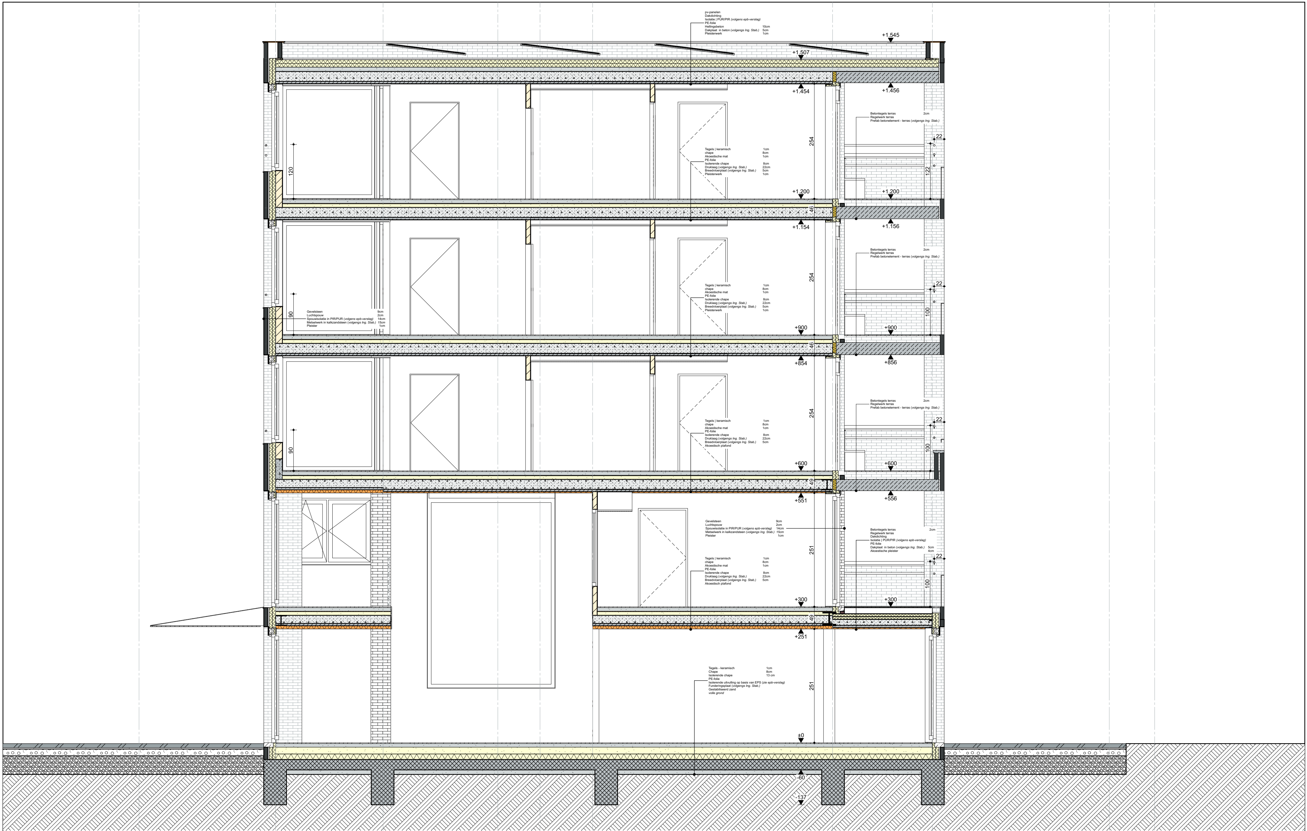
Doorsnede G-G NT
