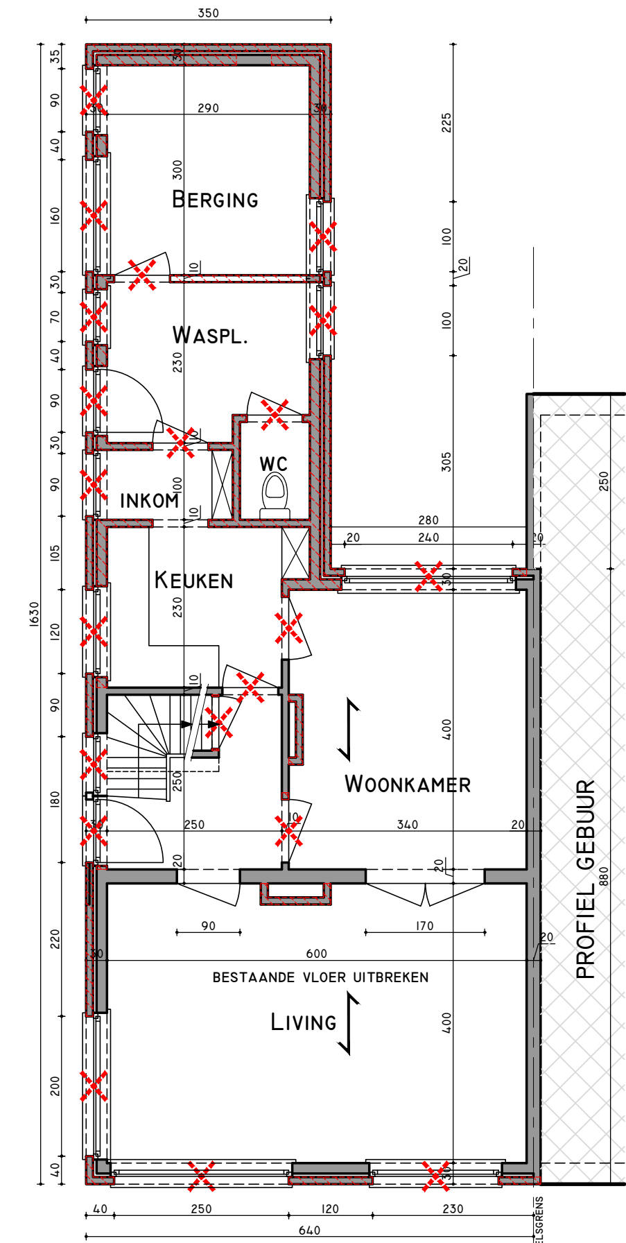
GRONDPLAN (0.00) - BESTAAND
