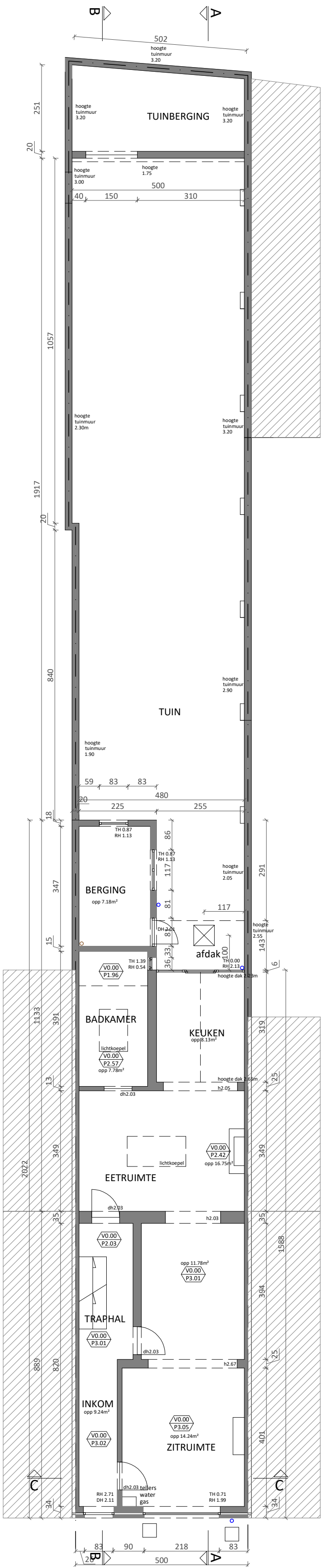
BESTAANDE TOESTAND GELIJKVLOERS 1-100
