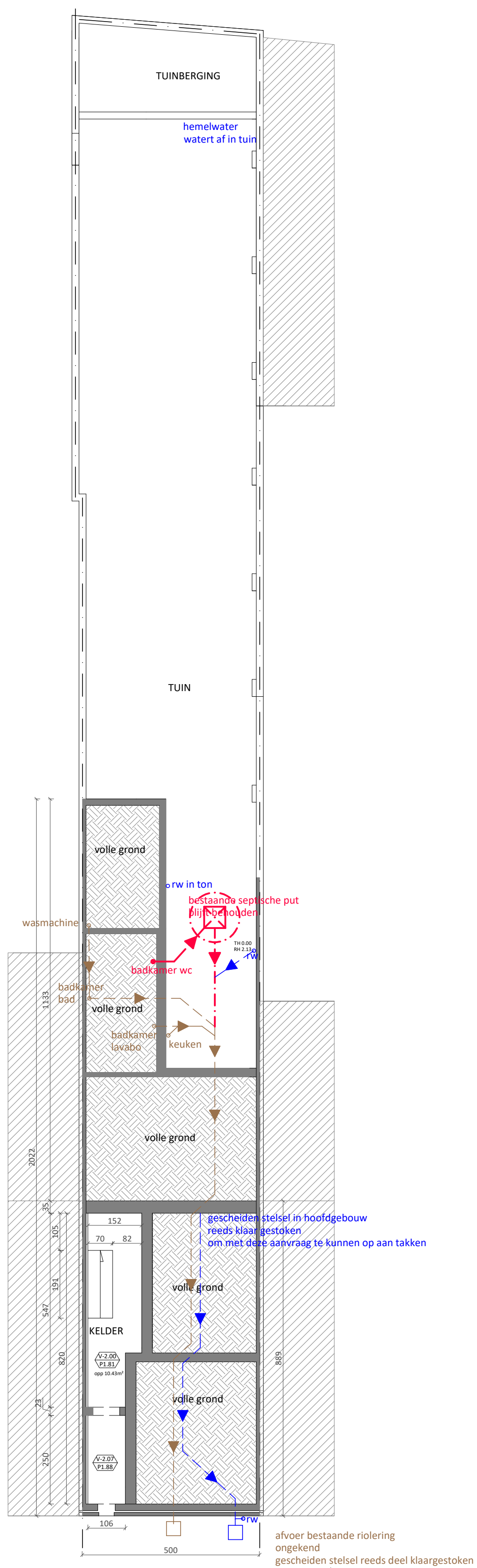
BESTAANDE TOESTAND KELDER 1-100 FUNDERINGS- en RIOLERINGSSHEMA
