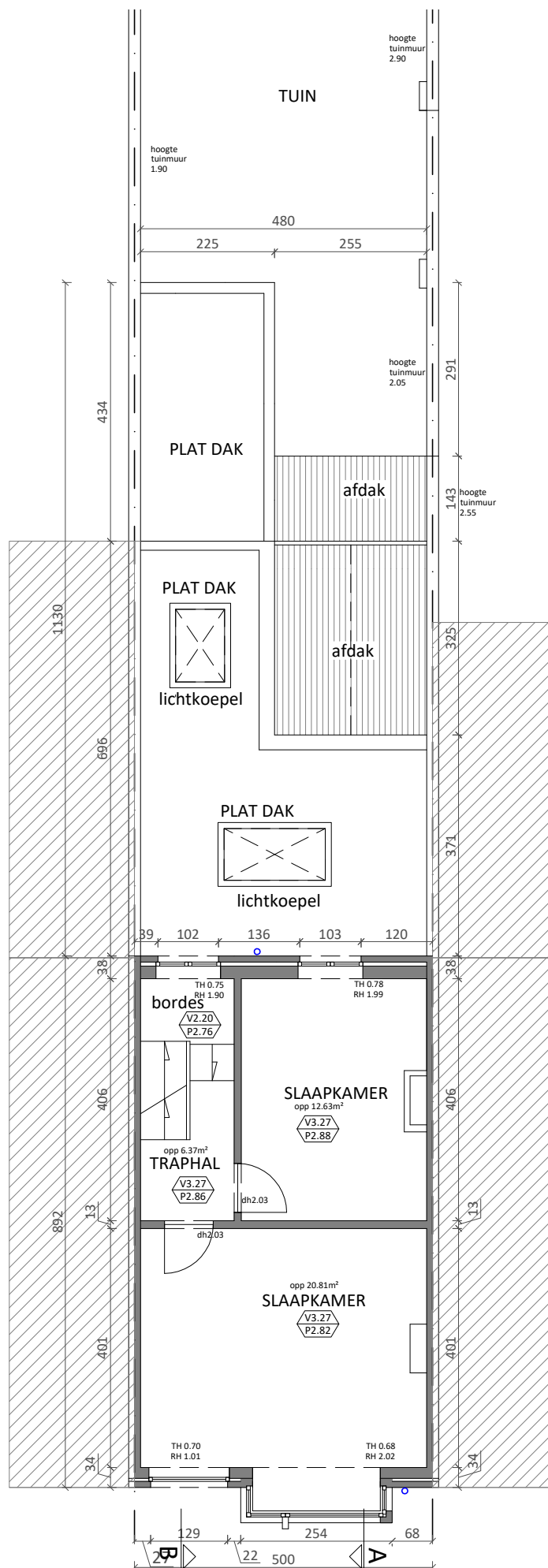
BESTAANDE TOESTAND EERSTE VERDIEP 1-100
