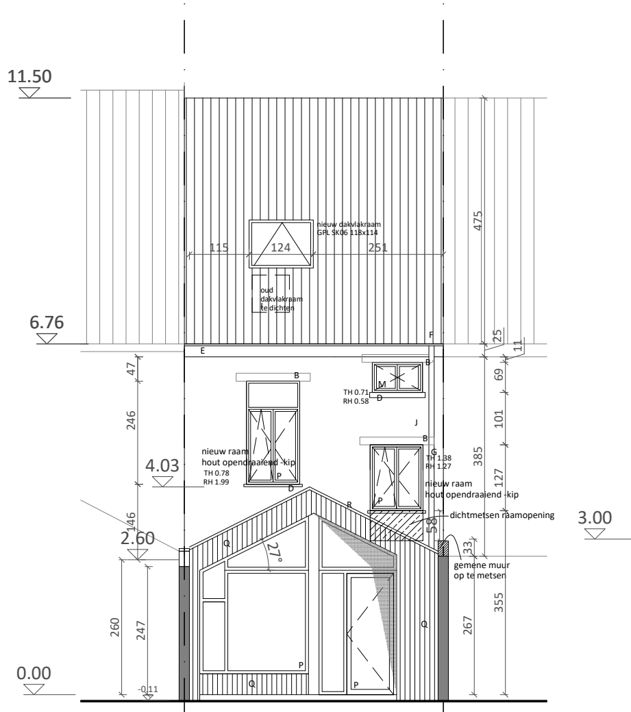
NIEUWE TOESTAND ACHTERGEVEL schaal 1-100
