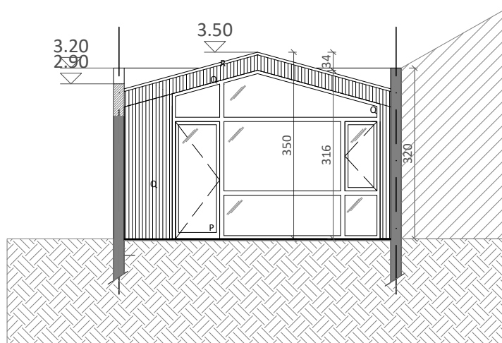
NIEUWE TOESTAND GEVEL TUINATELIER schaal 1-100
