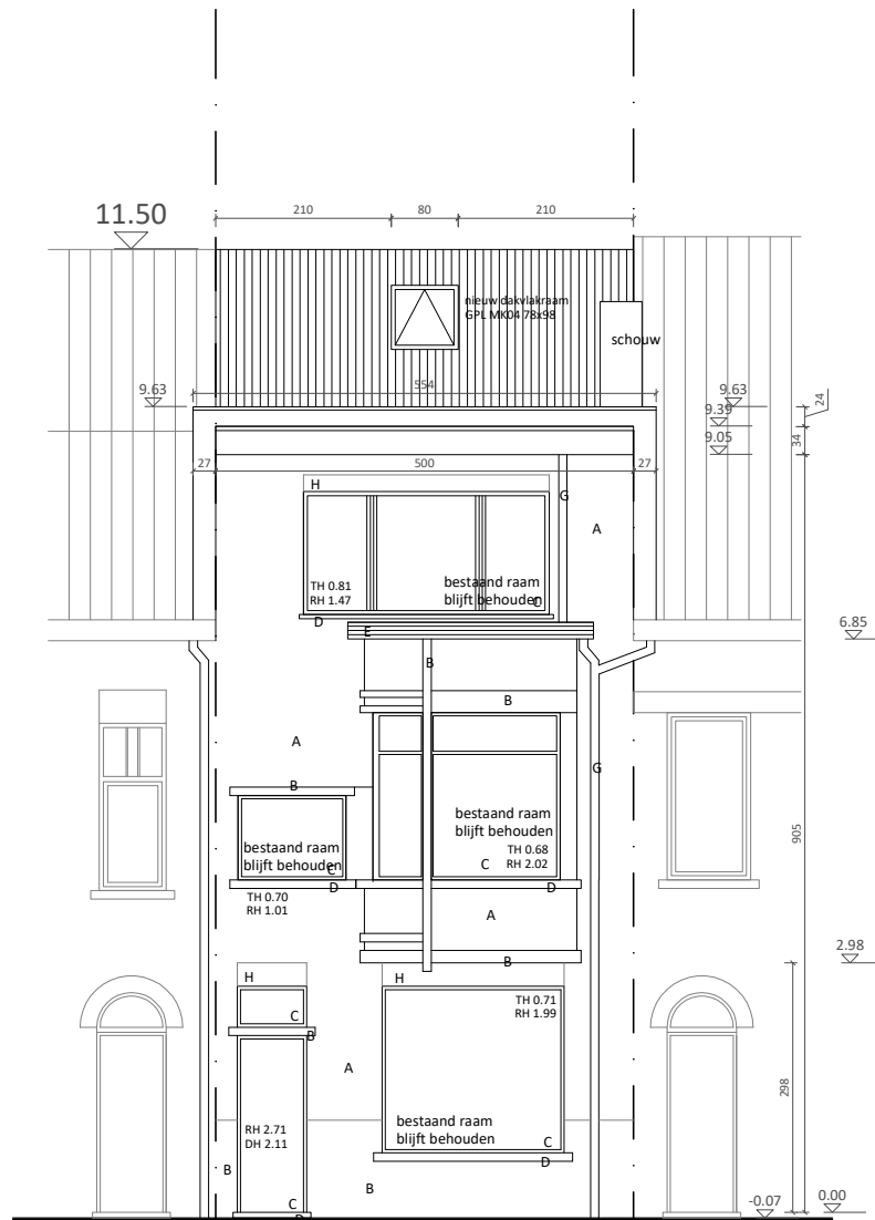
NIEUWE TOESTAND VOORGEVEL schaal 1-100
