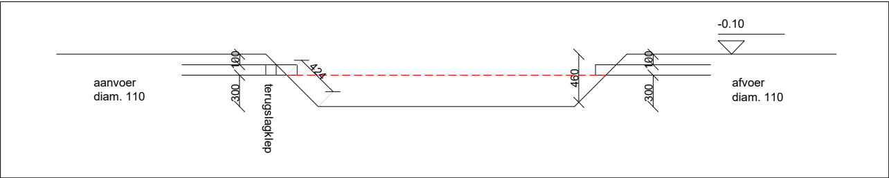
Detail infiltratievoorziening - schaal 1/50
