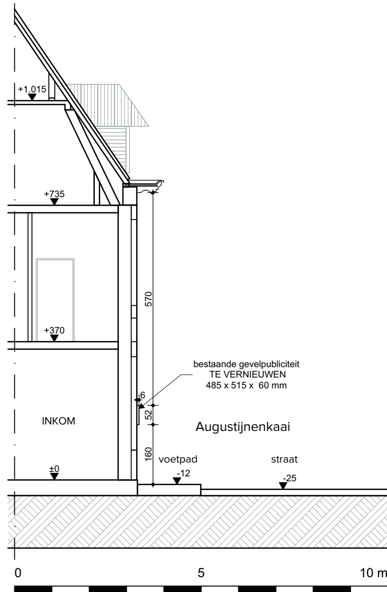
S DOORSNEDE - Bestaande toestand 1:100
