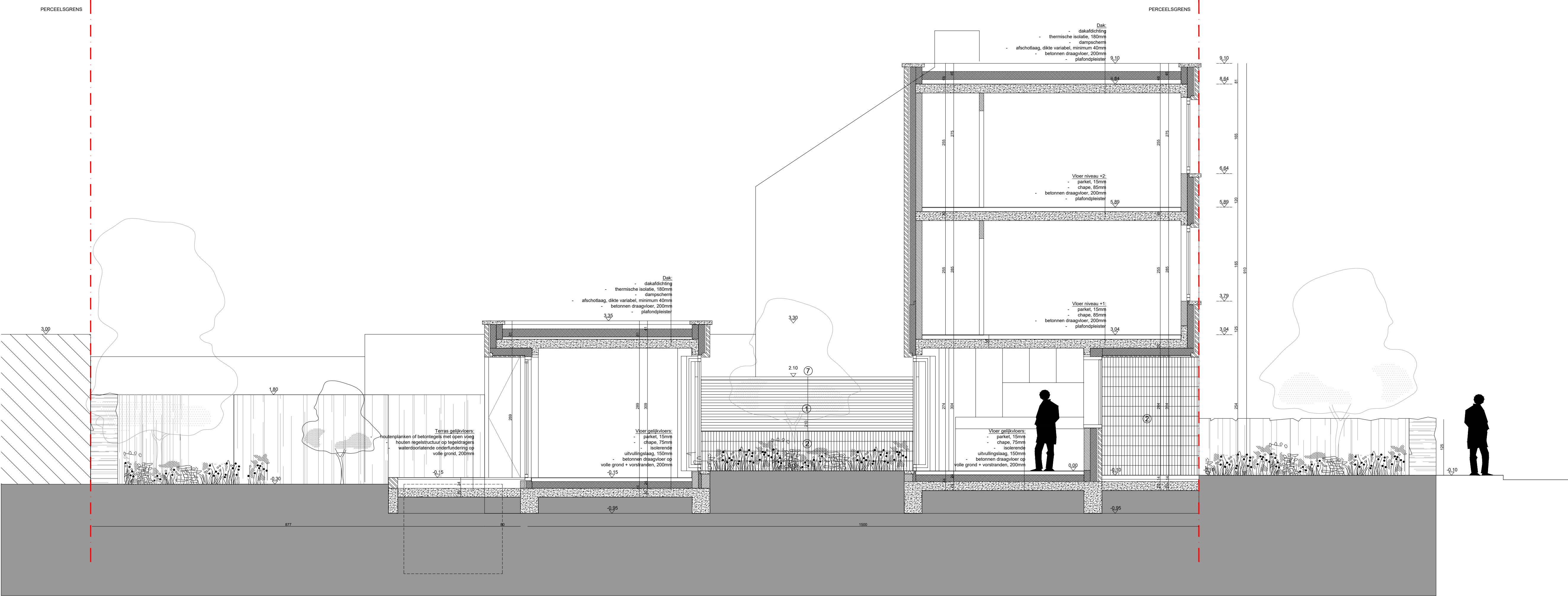
DOORSNEDE A2
