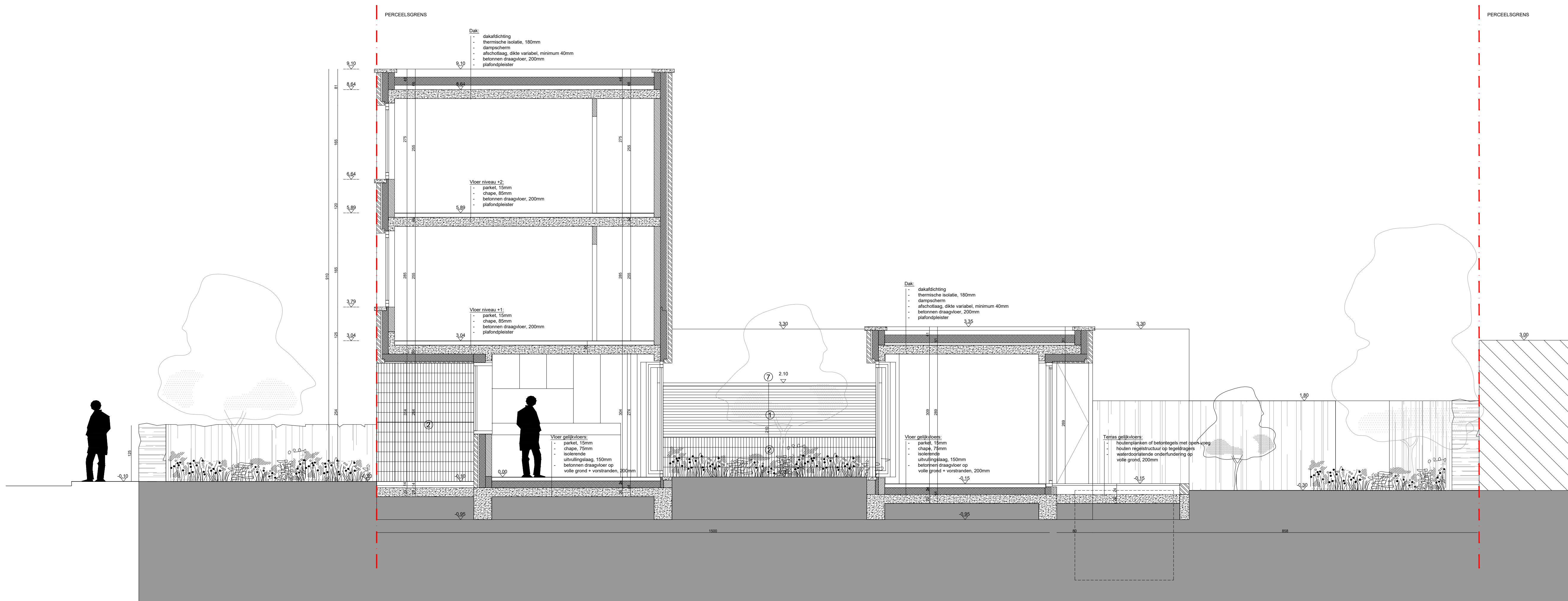
DOORSNEDE A1
