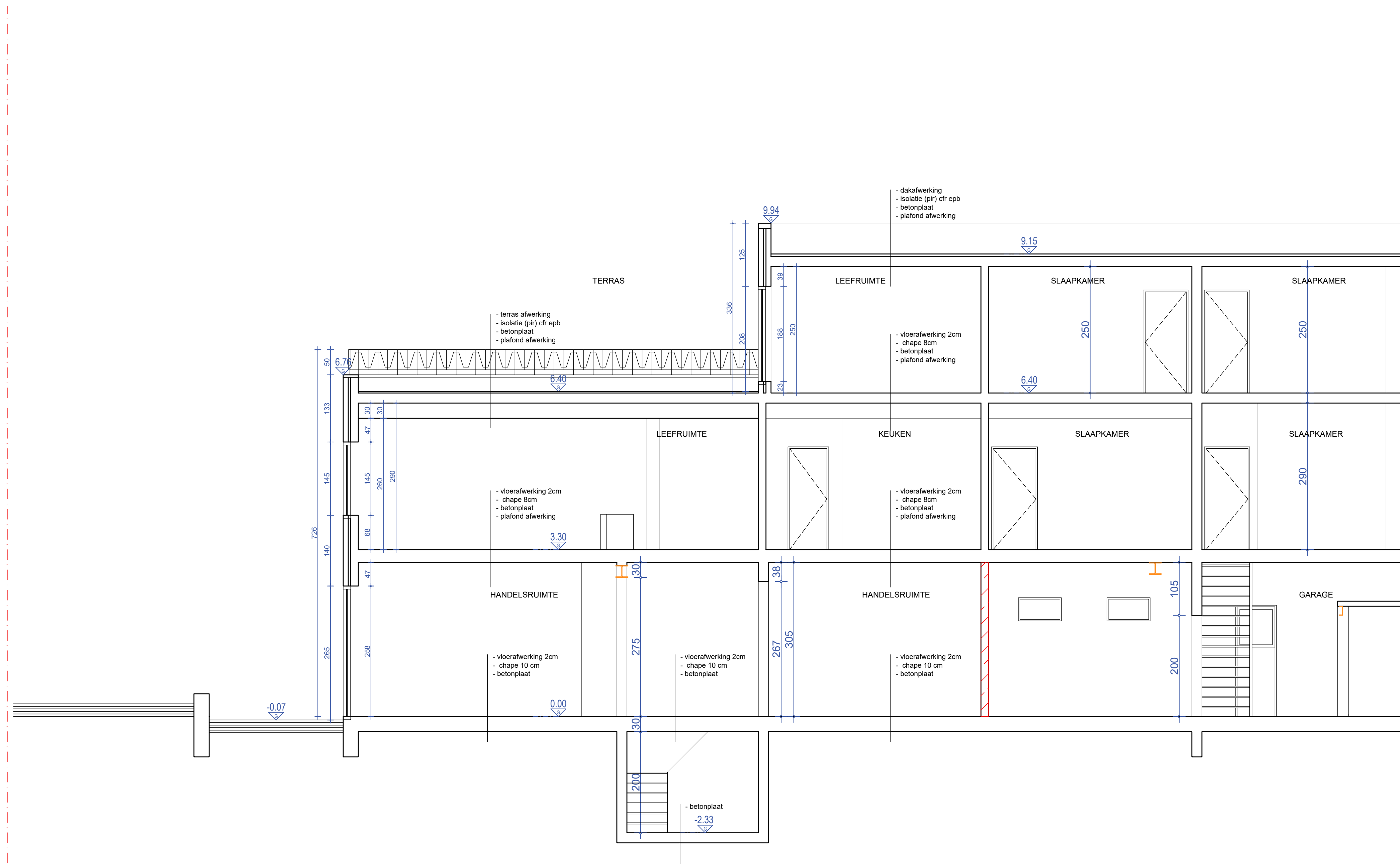
Principe snede BESTAANDE TOESTAND
