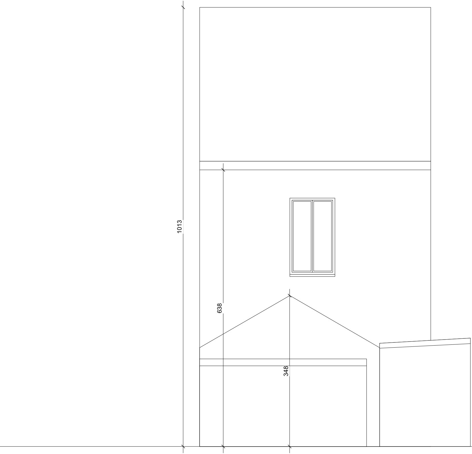
ACHTERGEVEL schaal 1/50
