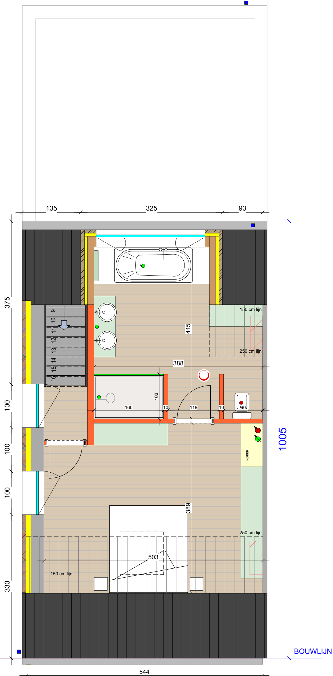
PLAN ZOLDER schaal 1/50
