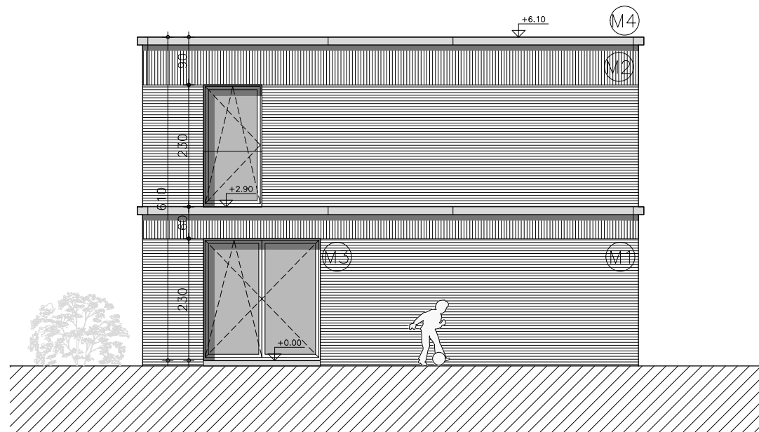
LOT 1 - ZIJGEVEL (NOORDOOST)
