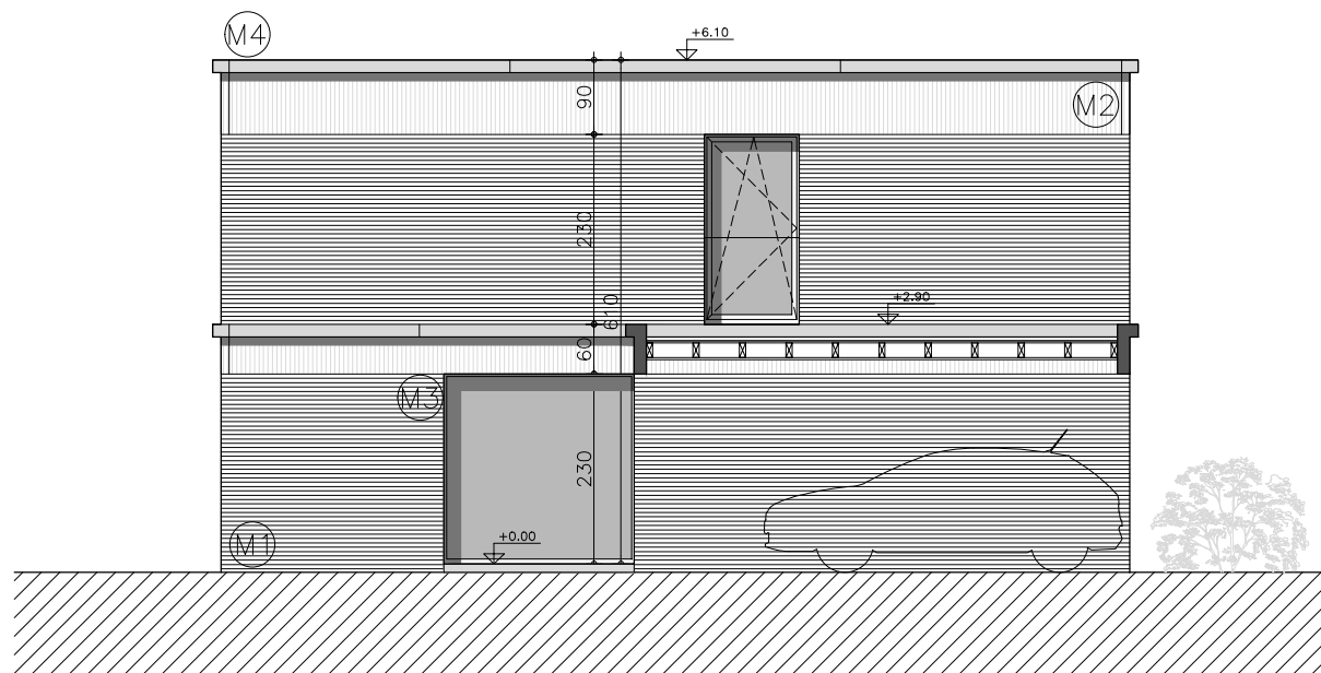
LOT 3 - ZIJGEVEL (NOORDOOST)
