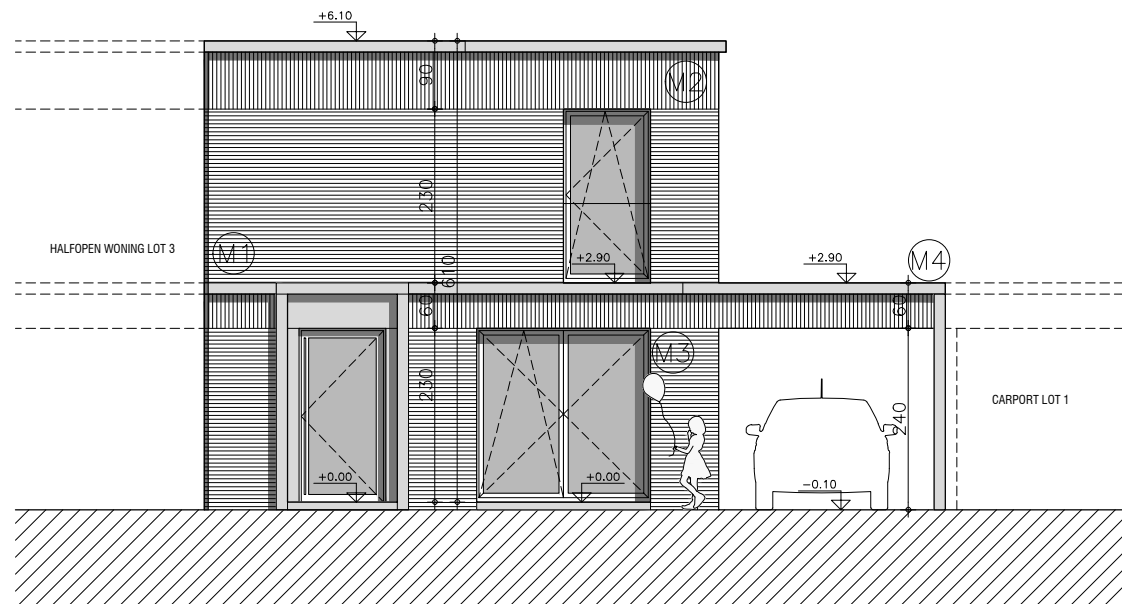
LOT 2 - VOORGEVEL (ZUIDOOST)
