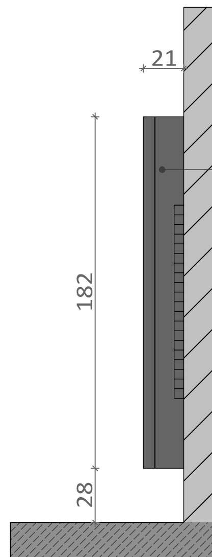
ZIJAAANZICHT
