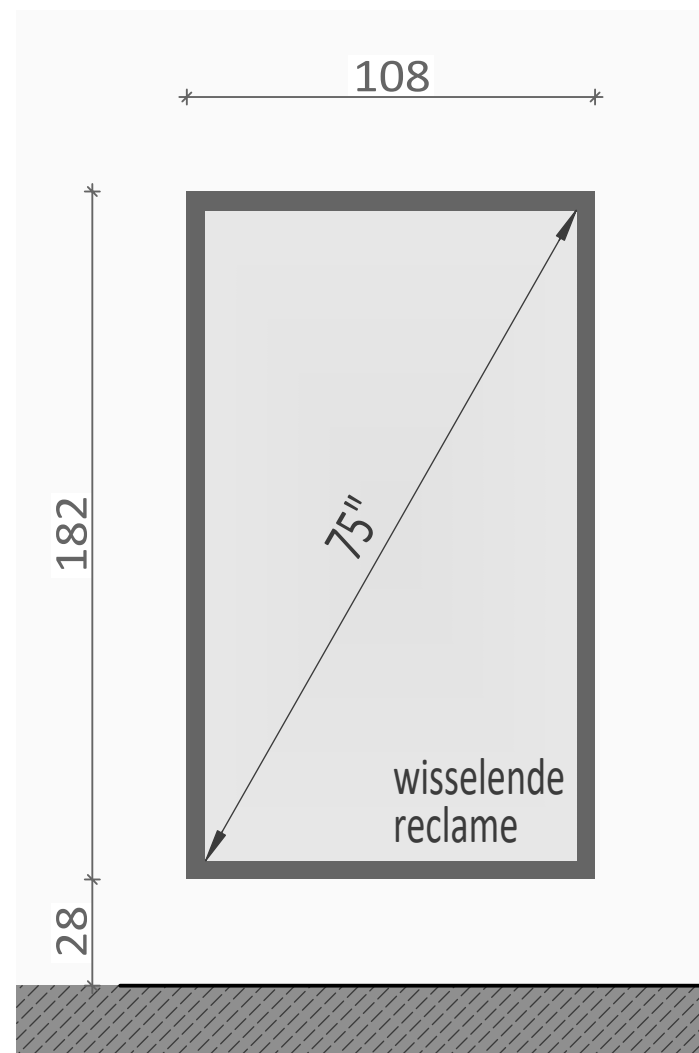
VOORAANZICHT
